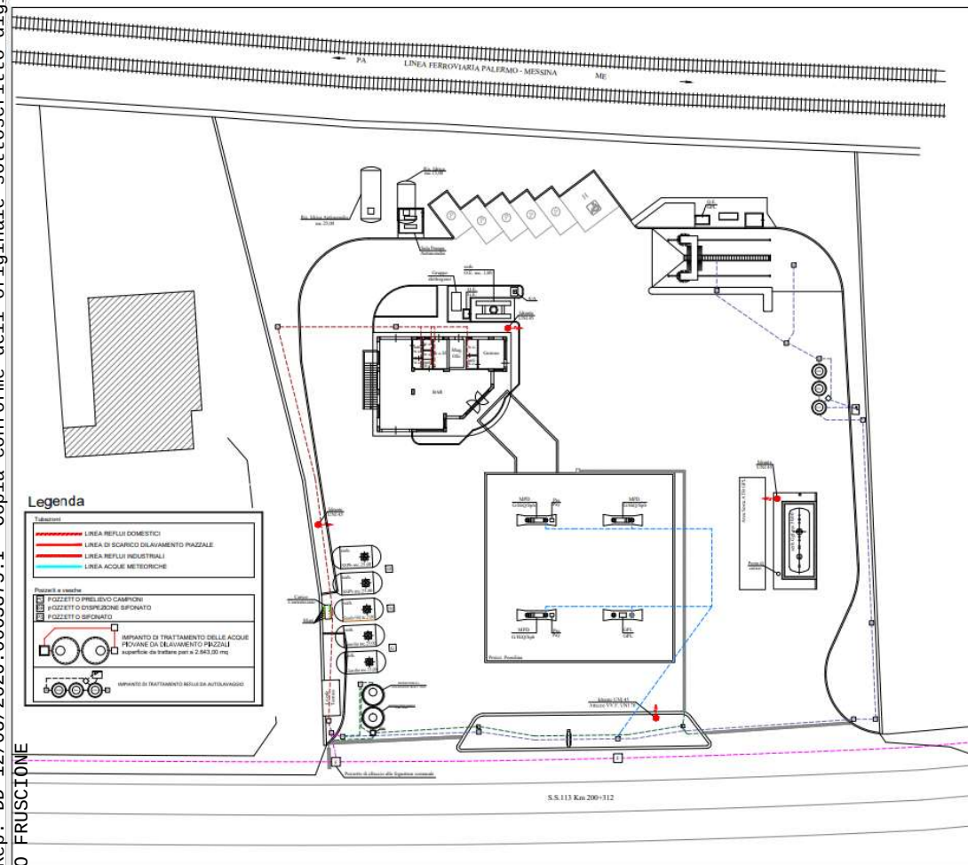
Planimetria stato di progetto - scala 1:200
