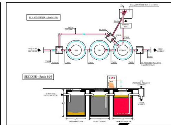
Particolare dimensionamento impianto di trattamento acque lavaggio - scala 1:50
