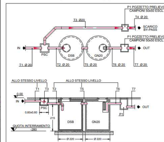
Particolare dimensionamento impianto di trattamento acque piazzale - scala 1:50
