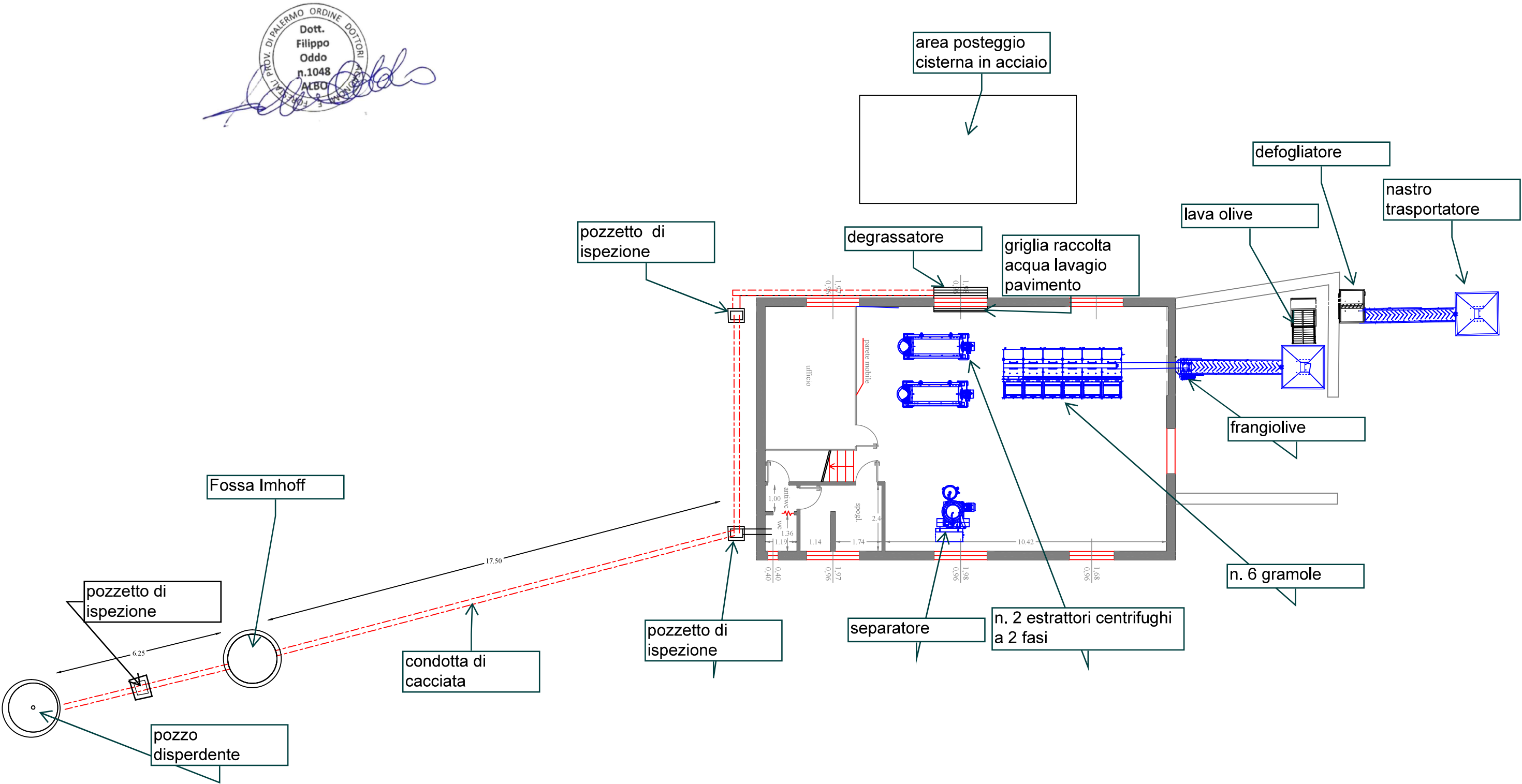
Planimetria con schema di allaccio fognario
